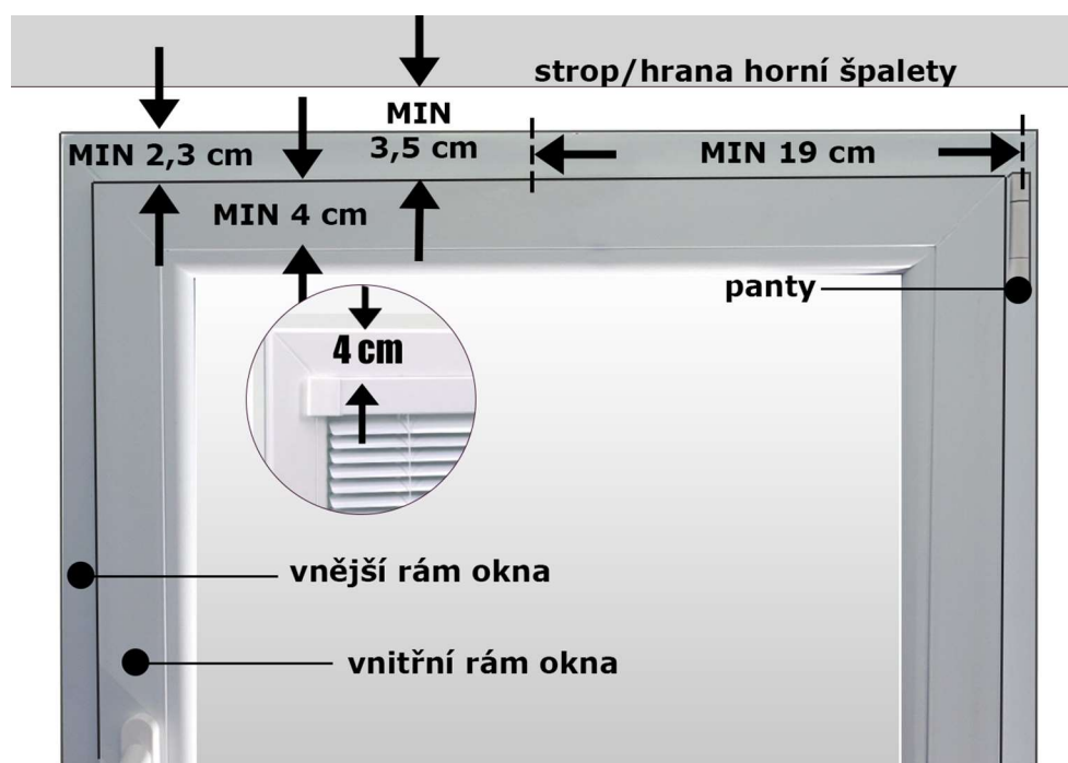
Obrázek #2A : Minimální požadavky na rozměry okna
